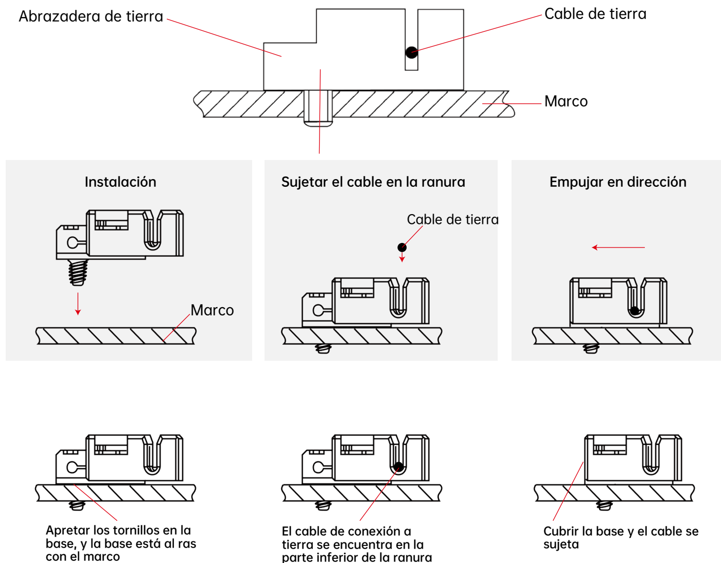
Figura 6 Modo de instalación del accesorio de puesta a tierra
