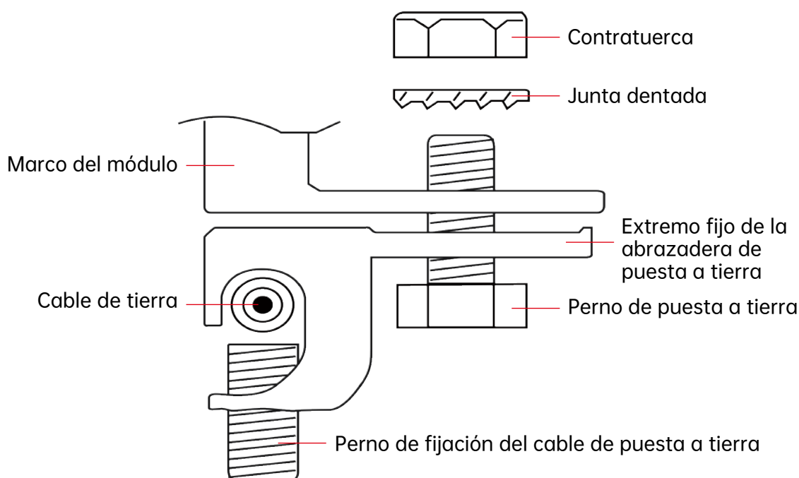
Figura 7 Método de instalación
