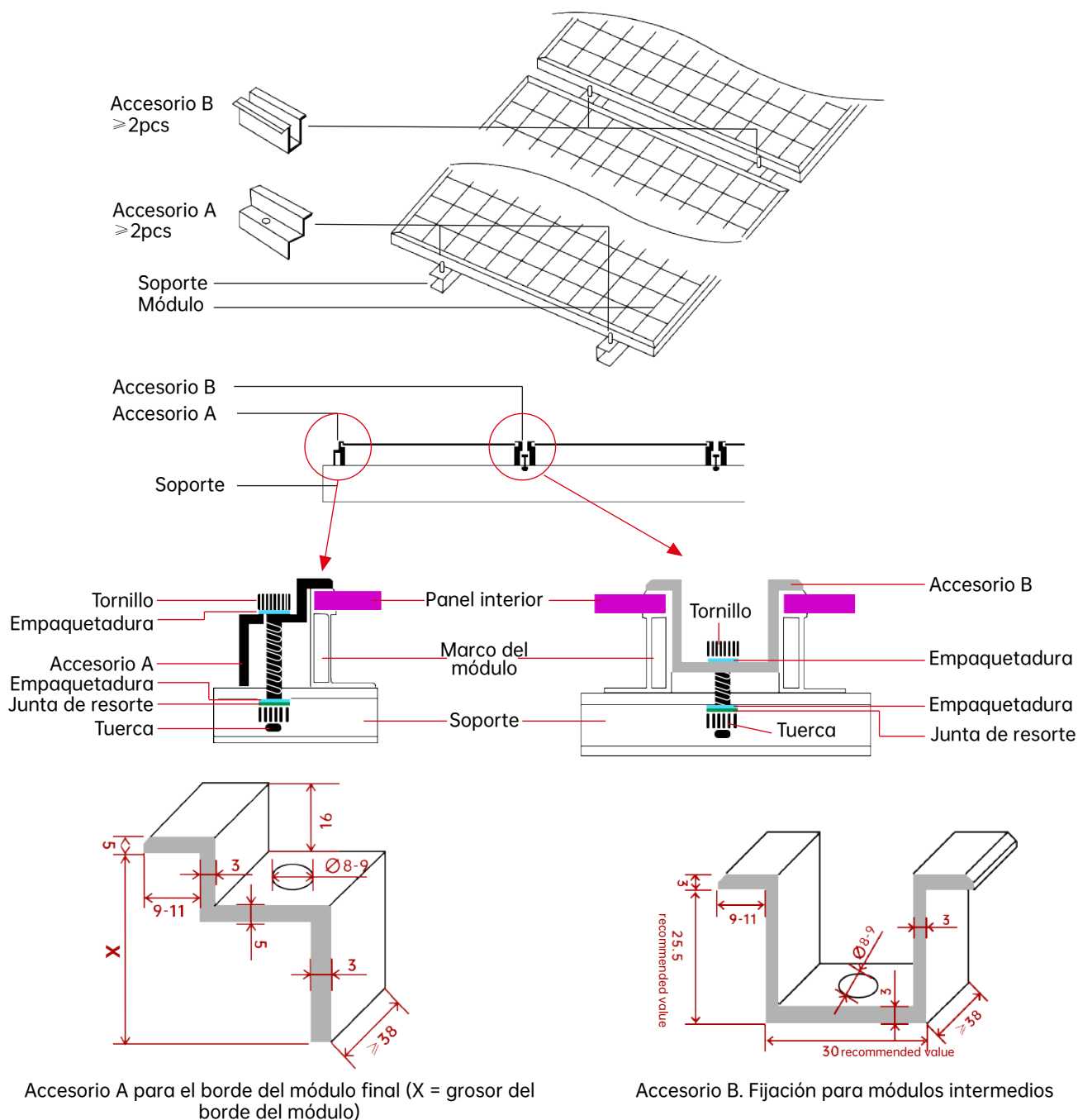
Fig. 3 Diagrama de accesorio (Unidad: mm)
